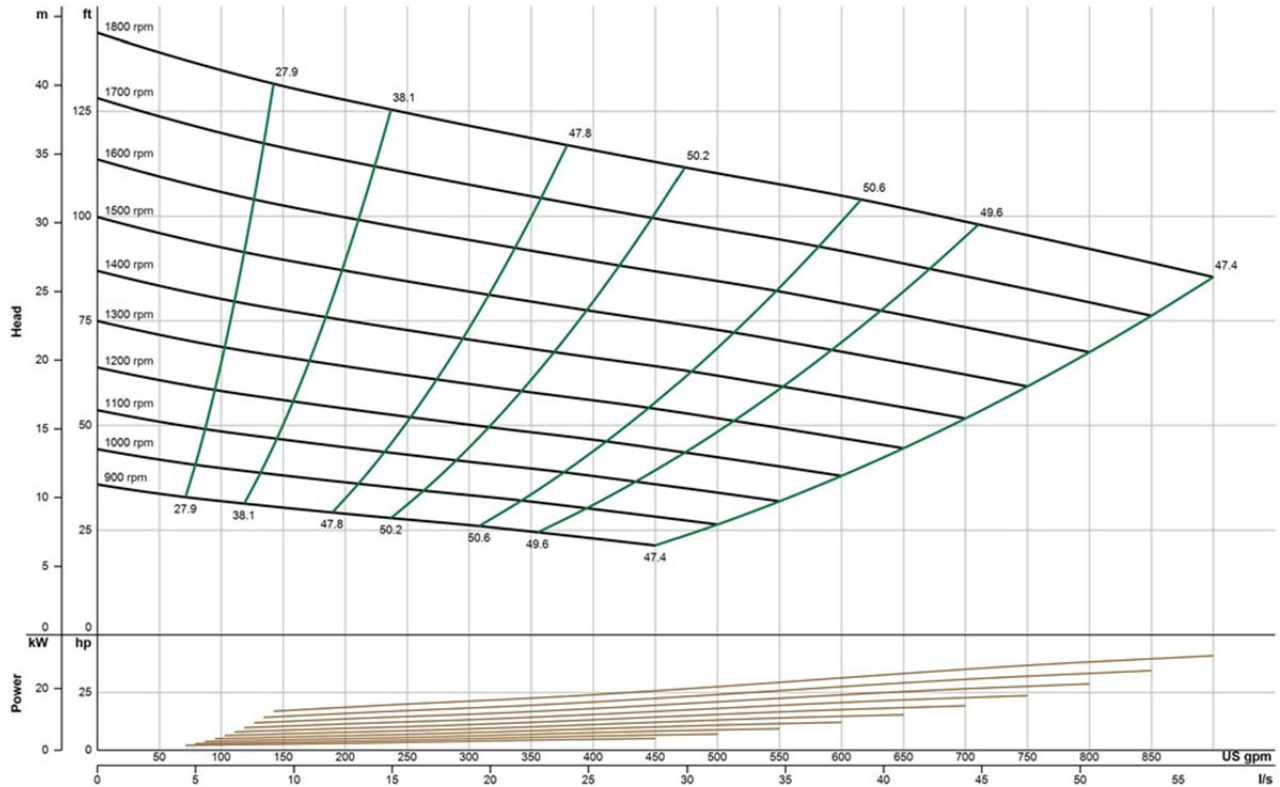
EDDY Pump - 3 Inch HD 3000 Curva de la Bomba de Lodo Líquido
